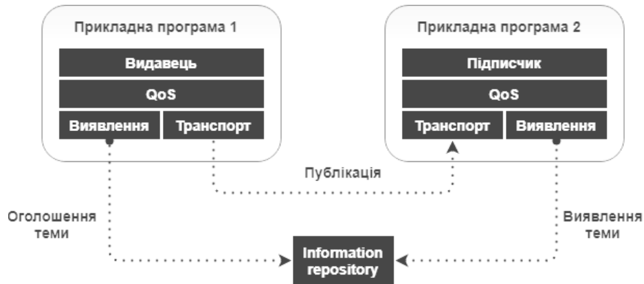
Рис. 4. Централізована взаємодія прикладних програм з DDS
